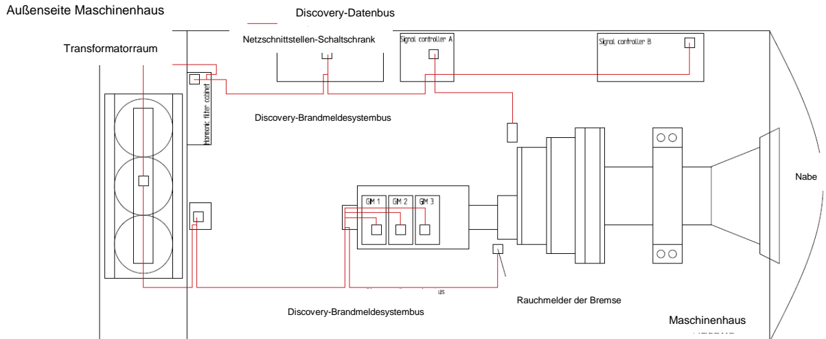
Abbildung 7-1: Beispiel für Systemaufbau in 2.0 MW, Mk 8
