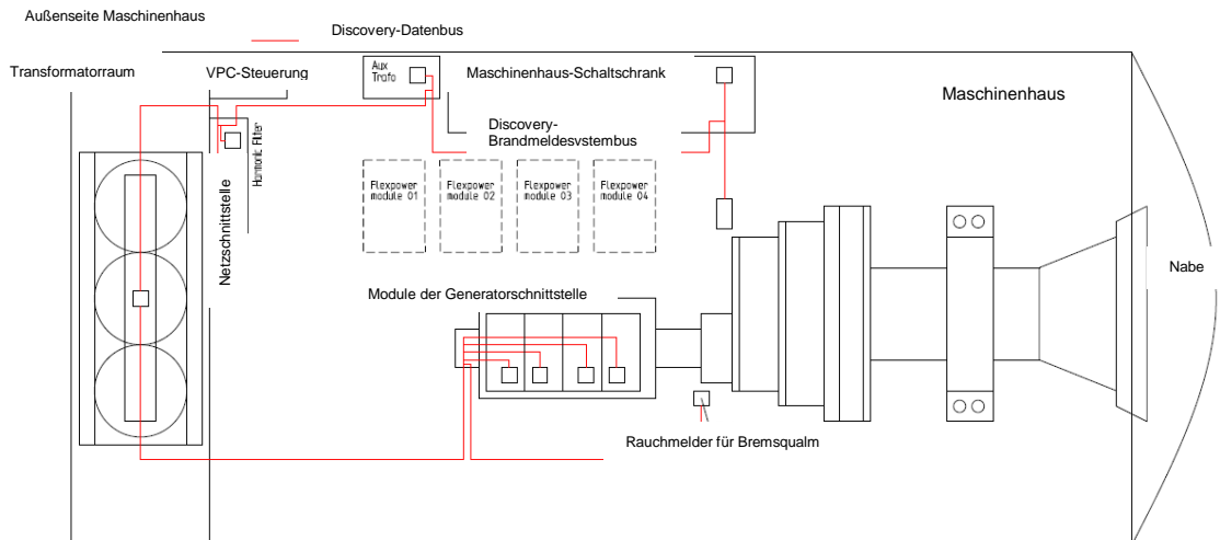
Abbildung 7-2: Beispiel für Systemaufbau in V112-3.0 MW
