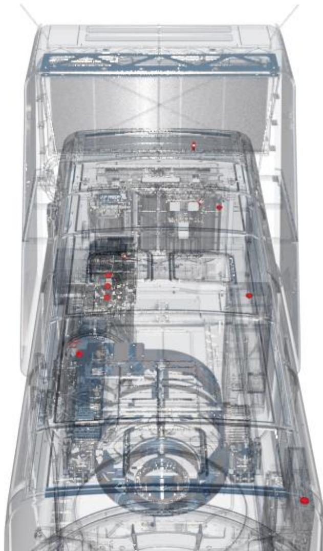
Abbildung 6-1: Rauchmeldeanlage (rot) im Maschinenhaus (2.0 MW, Mk 8 wird als Beispiel verwendet)
