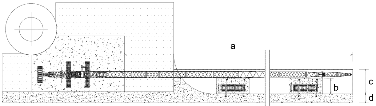
Abb. 13: Kranauslegermontagefläche
