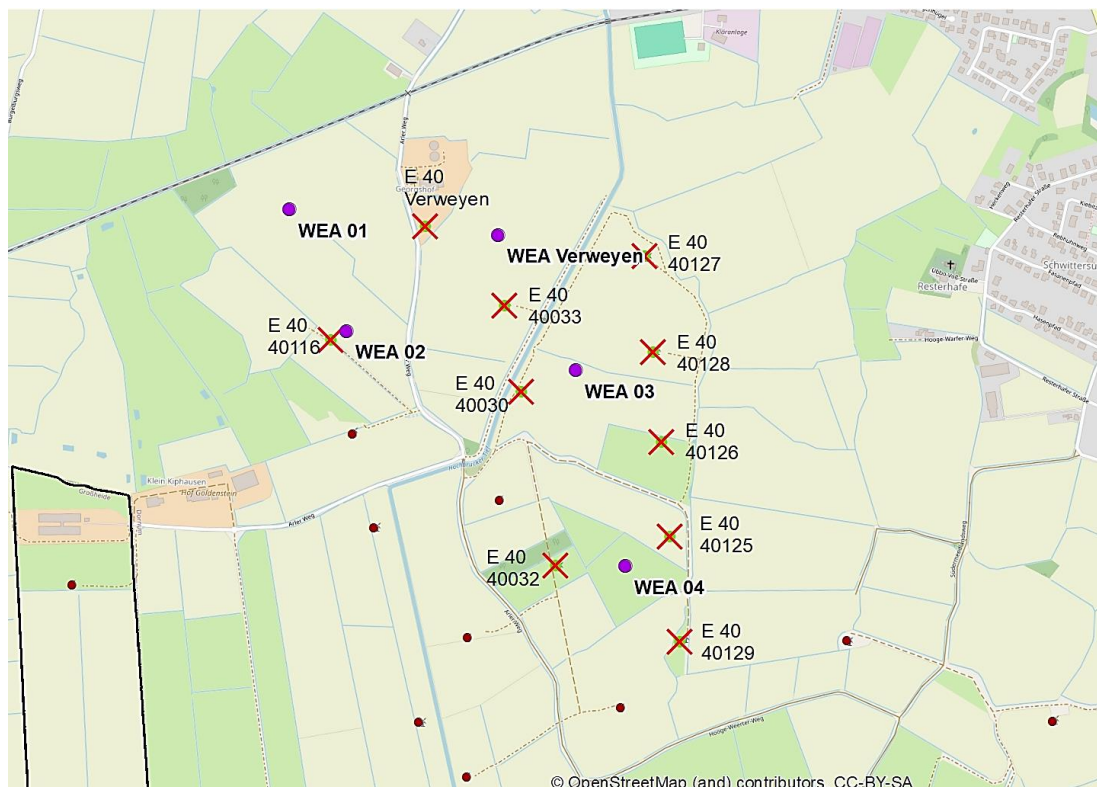
Abb. 13: Detailansicht zur räumlichen Lage der Repowering-Maßnahme
