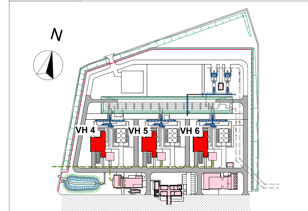
Übersichtsplan
