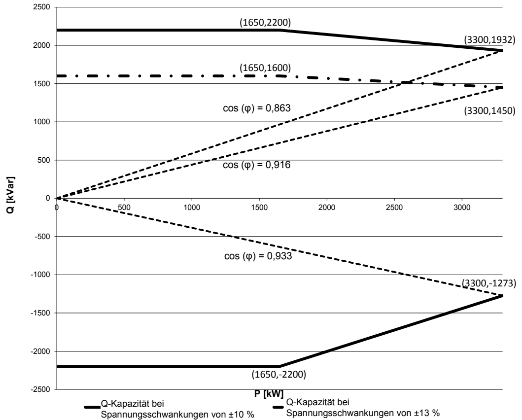
Abbildung 9-3: Blindleistungskapazität bei 3,3-MW-Bemessungsleistung
