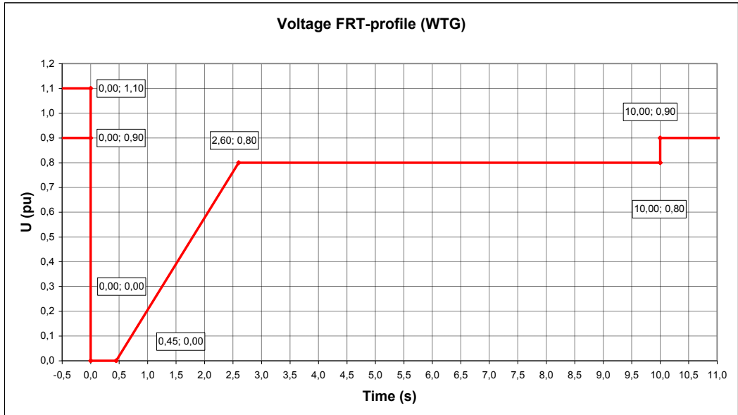
Abbildung 9-5: Niedrige Spannungstoleranzkurve für symmetrische und asymmetrische Störungen, wobei U die gemessene Spannung im Stromnetz darstellt
