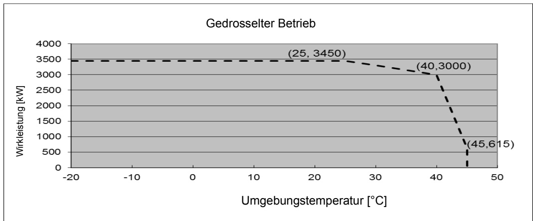
Abbildung 9-2: Heruntergeregelter Betrieb bei 3,45-MW-Bemessung
