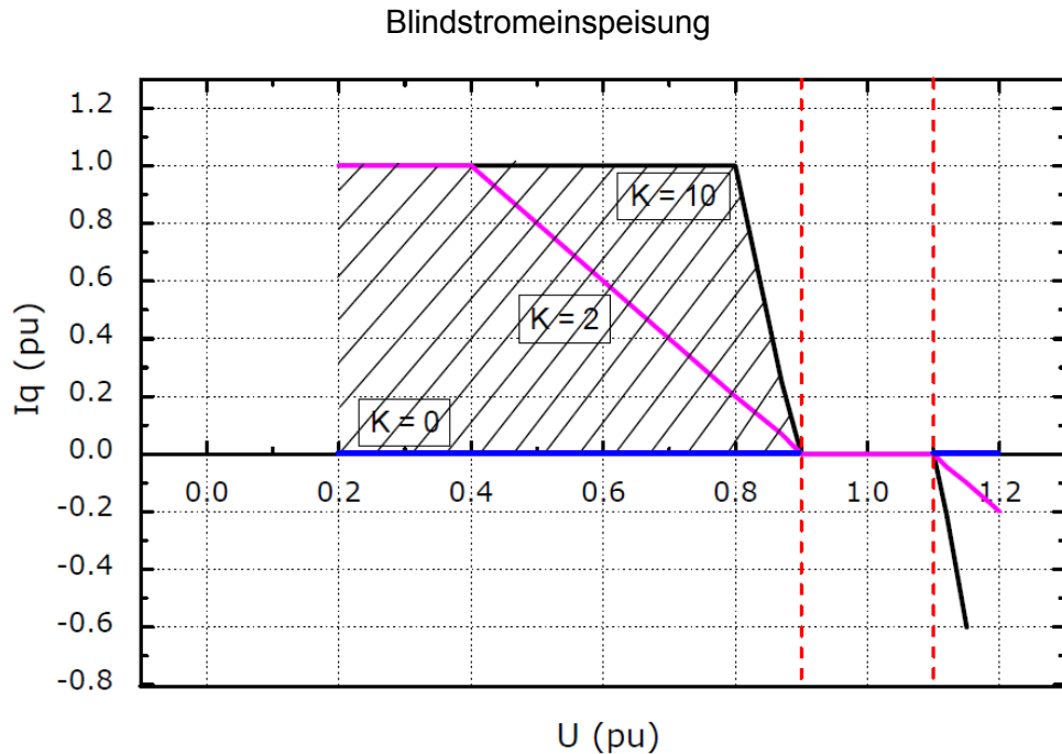
Abbildung 9-6: Blindstromeinspeisung
