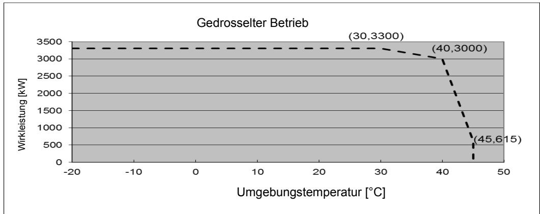
Abbildung 9-1: Heruntergeregelter Betrieb bei 3,3-MW-Bemessung
