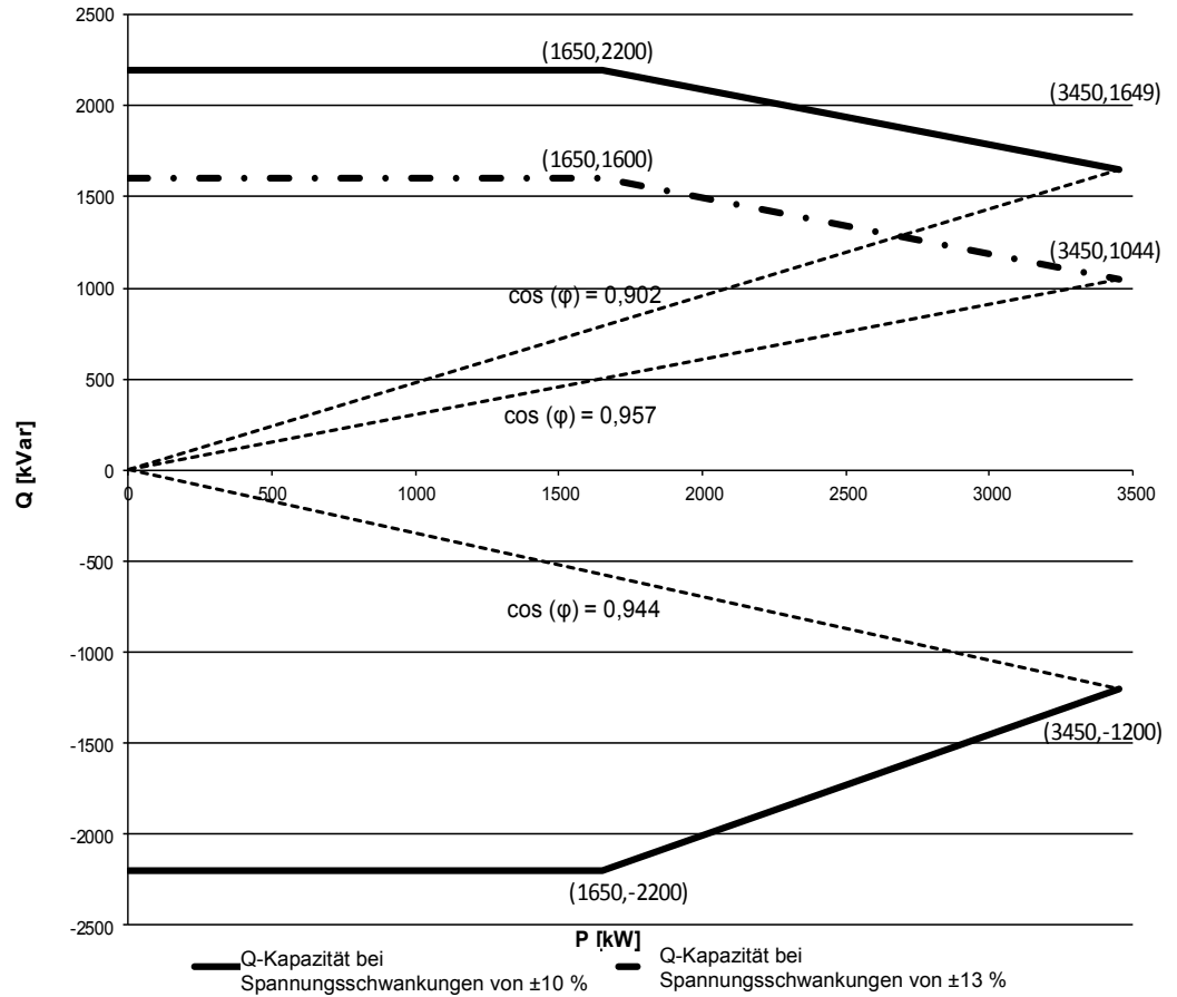
Abbildung 9-4: Blindleistungskapazität bei 3,45 MW Bemessungsleistung
