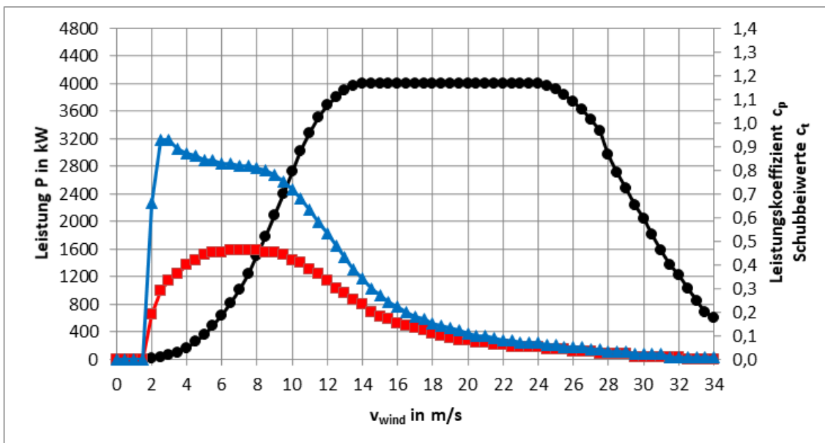
Abb. 2: Leistungs-, c_p - und c_t -Kennlinie E-115 EP3 E3 / 4200 kW Betriebsmodus I s
