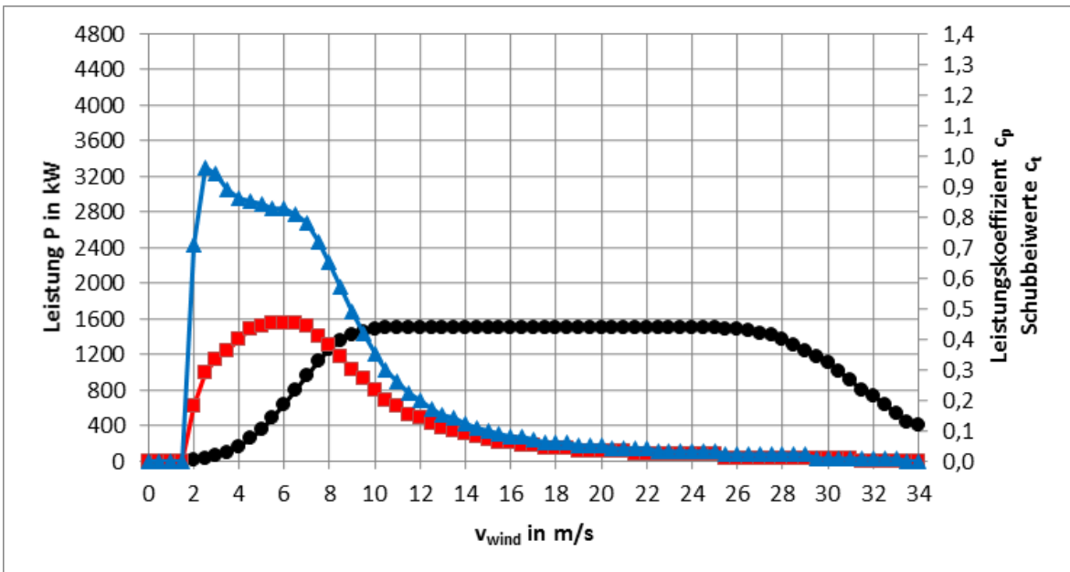
Abb. 8: Leistungs-, c_p - und c_t -Kennlinie E-115 EP3 E3 / 4200 kW Betriebsmodus 1500 kW s
