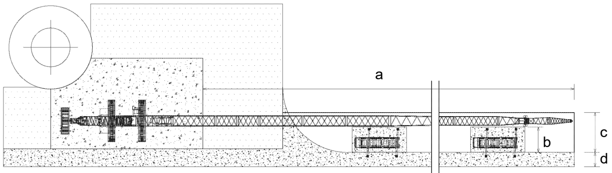
Abb. 13: Kranauslegermontagefläche
