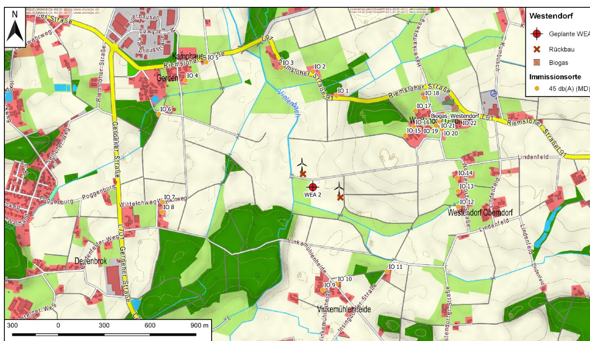
Abbildung 6.1: Lage der betrachteten Immissionsorte sowie der WEA-Standorte am Standort Westendorf
