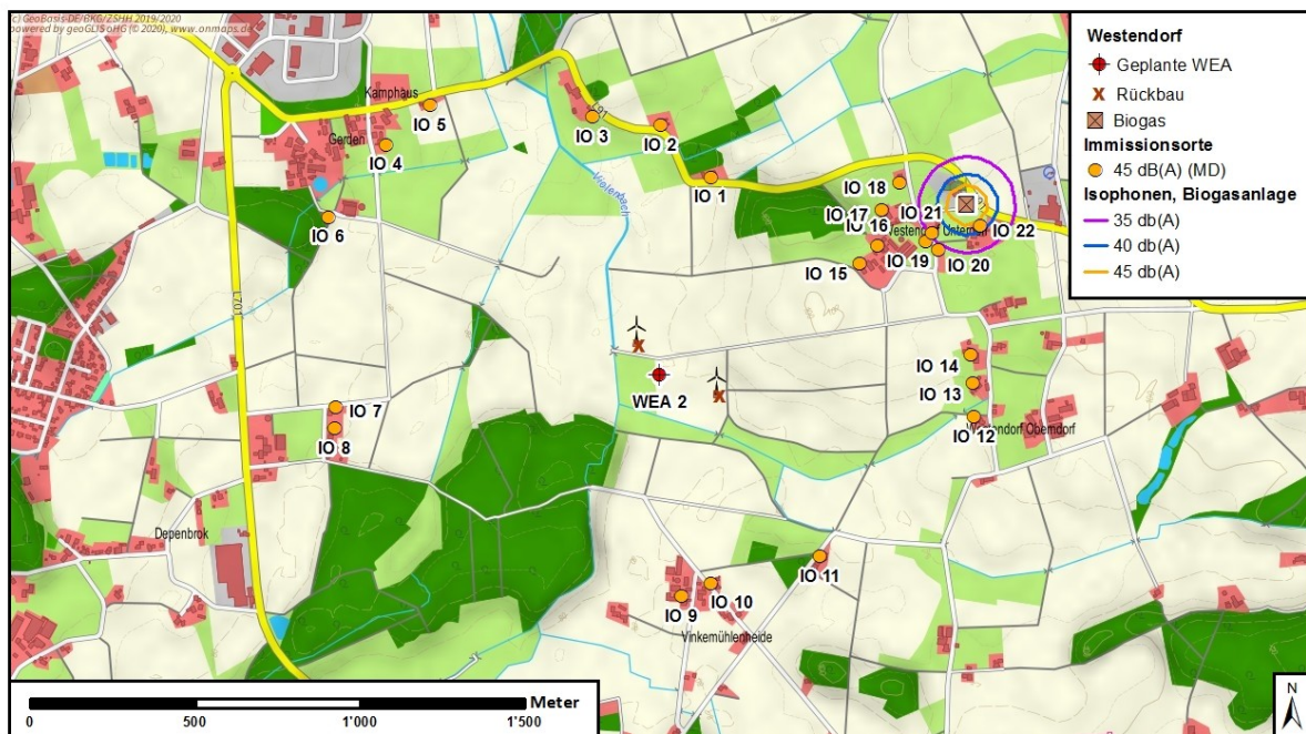
Abbildung D.1 : Isophonenkarte der Vorbelastung durch die Biogasanlage, ohne Berücksichtigung von Unsicherheiten
