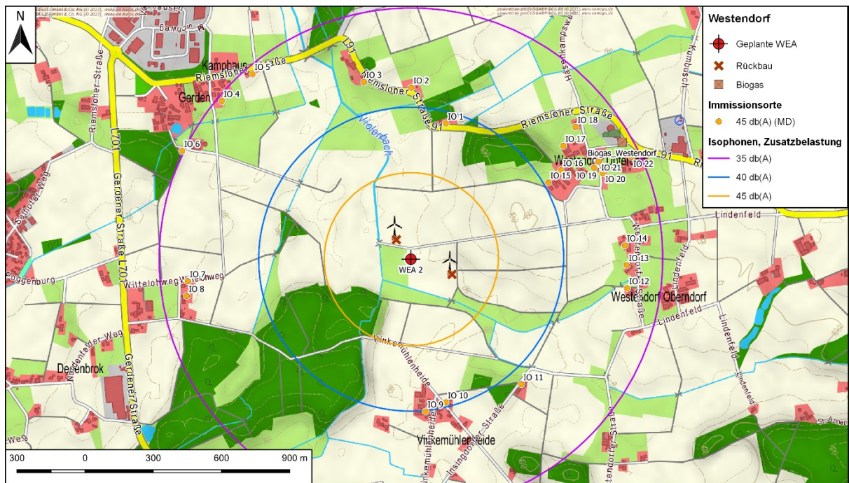
Abbildung D.2: Isophonenkarte der Zusatzbelastung, ohne Berücksichtigung von Unsicherheiten
