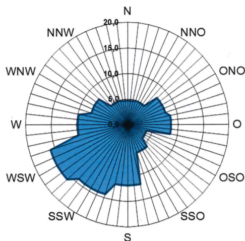
Abbildung 2: Relative Häufigkeit der Windrichtung am Standort Hollenstede (Fläche 17) in Prozent (Bezugshöhe 159,64m ü. Grund) /22/
