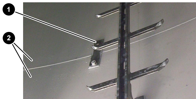
Abb. 10: Überbrückungslasche zwischen 2 Betonfertigteilstegmenten
