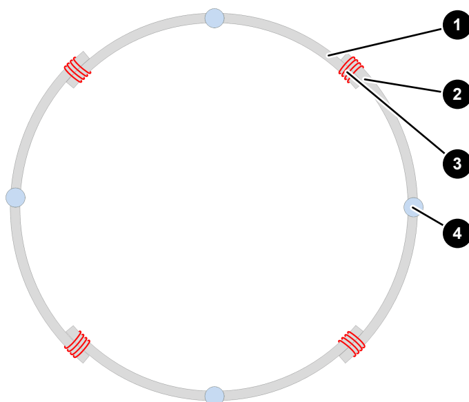
Abb. 11: Nutzung der Bewehrung als Ringleiter im Betonfertigteilstegment
