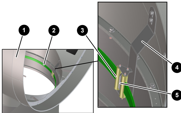
Abb. 6: Ableitring am Blattanschluss mit Rollenblitzableiter am Beispiel der E-82 E2
