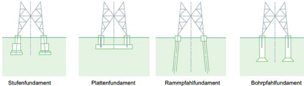
Abbildung 2: Schematische Darstellung von Grundungstypen.
