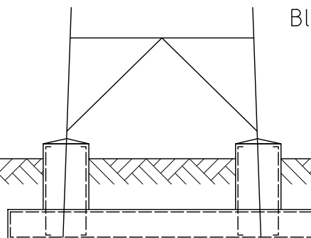
Plattenfundament
