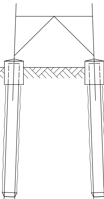
Rammgründung (Rohr ummantelt)
