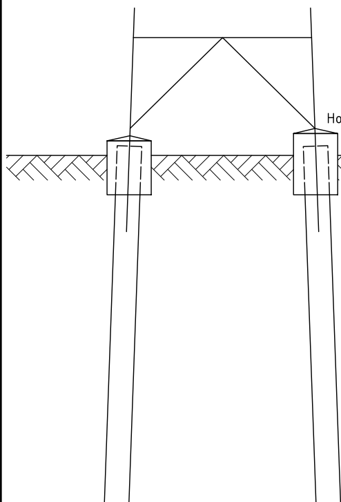
Rammgründung (Rohr unbeschichtet)
