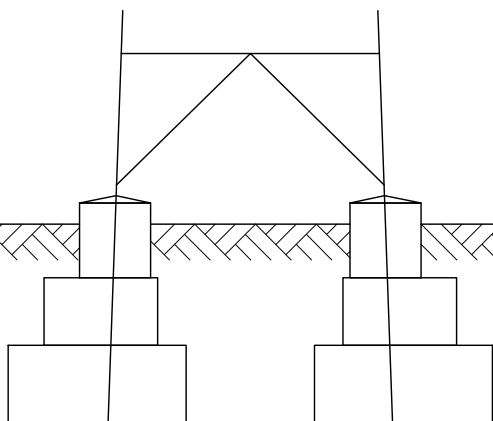
Stufenfundament
