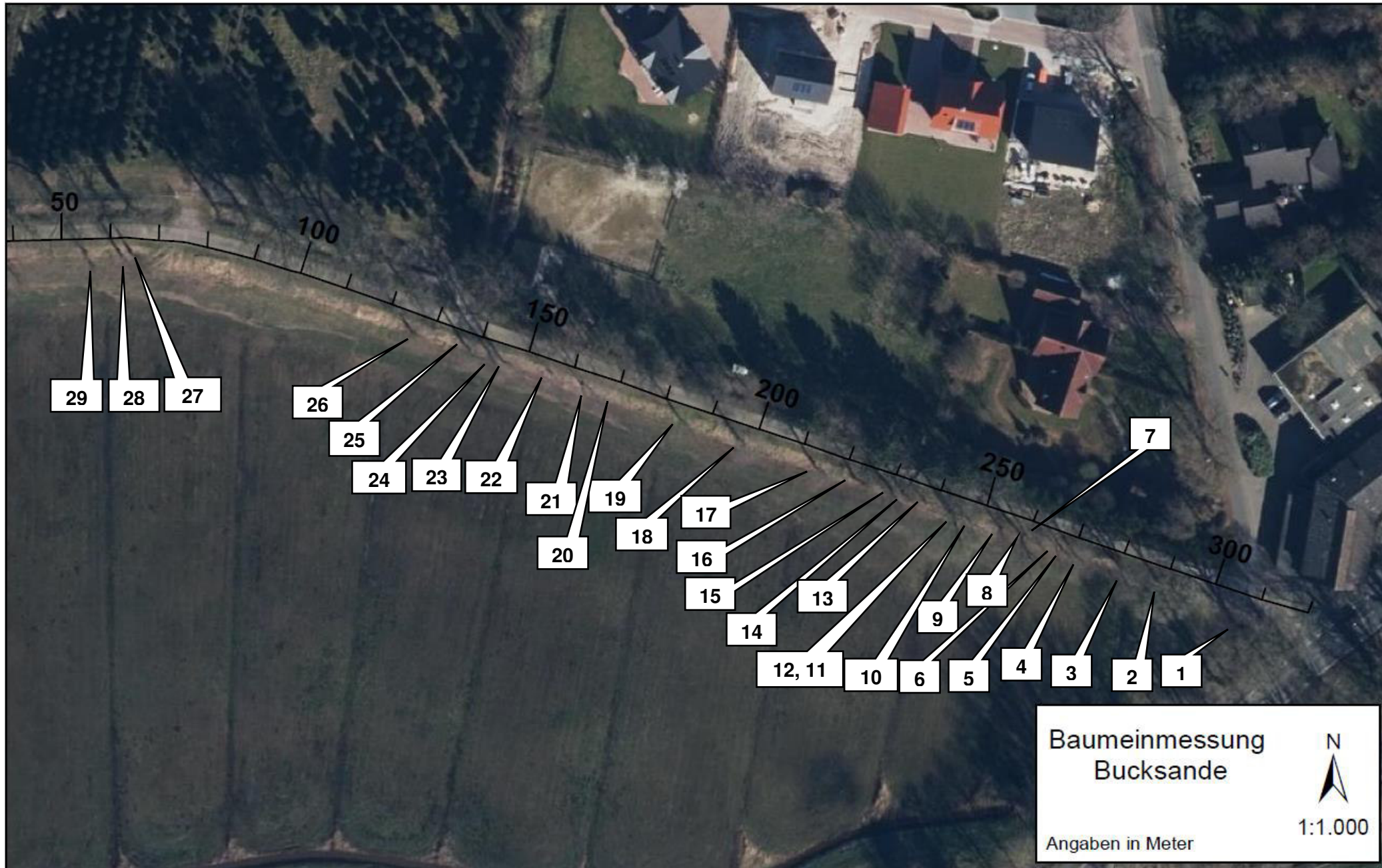
Anlage 14.3 Baumeinmessung
