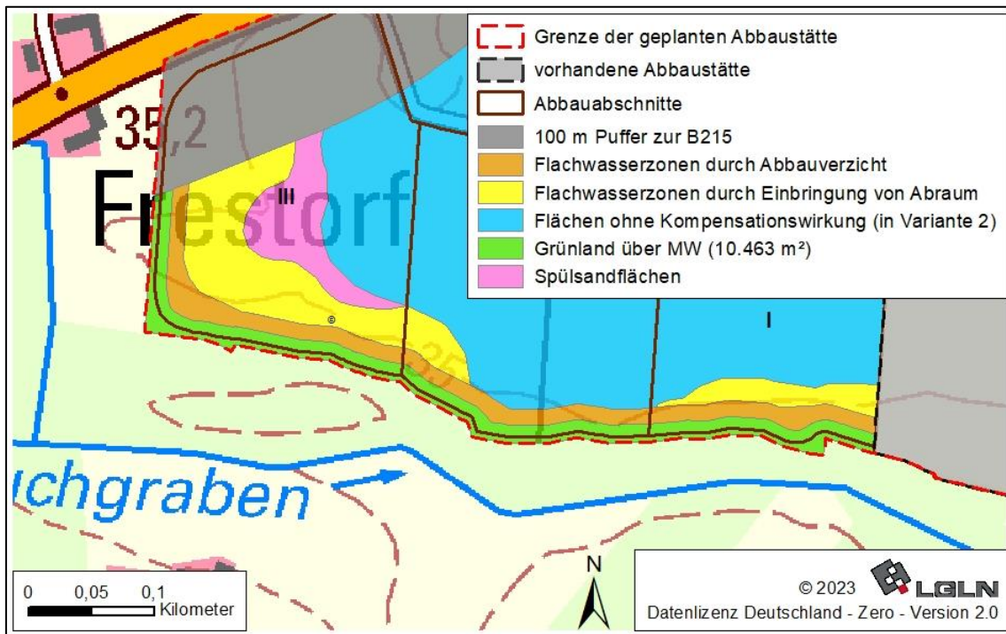
Abb. 7 Detailplan zur Flächenermittlung zur Rahmenvereinbarung Wesertal
