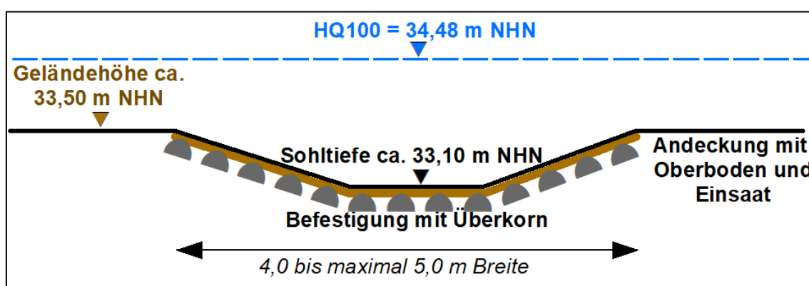
Abb. 4 Prinzipskizze Hochwasserüberlauf
