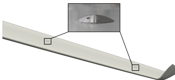
Abb. 3: Rotorblatt mit Rezeptoren auf der Druck- und Saugseite
