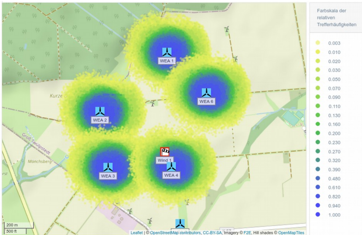
Abbildung A.1.1: Trefferhäufigkeiten von Eisstücken pro Rasterfläche (16m 2 ) und Jahr in der Umgebung der WEA 1 - 4 und 6 am Standort Volkmarsdorf (Karte 171).
