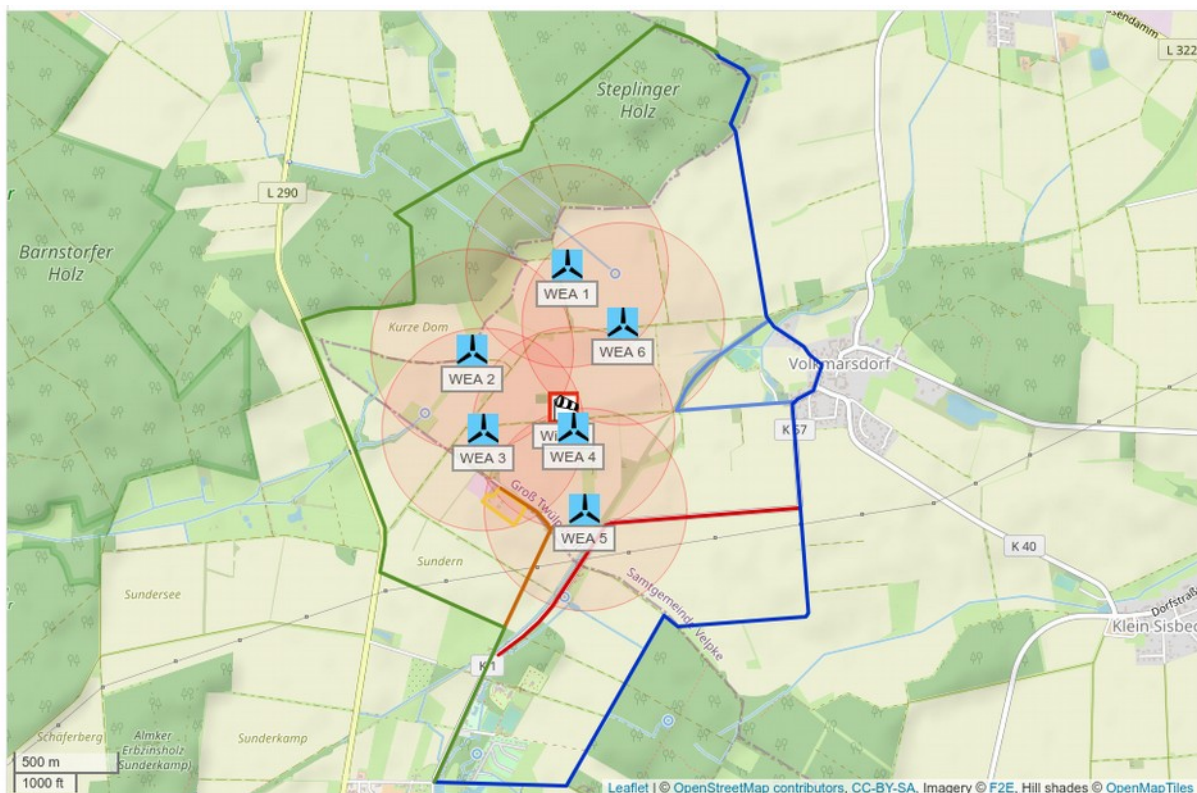
Abbildung 4.3.1: Potentielle Gefährdungsbereiche der WEA 1 - 6 und Schutzobjekte am Standort Volkmarsdorf (Karte 171).
