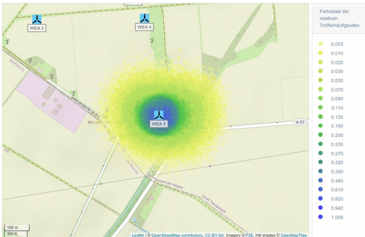
Abbildung B.1.1: Trefferhäufigkeiten von Eisstücken pro Rasterfläche (16m 2 ) und Jahr in der Umgebung der WEA 5 am Standort Volkmarsdorf (Karte 171).
