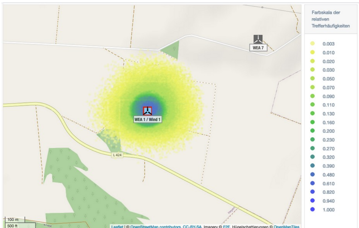
Abbildung B.1.1: Trefferhäufigkeiten von Eisstücken pro Rasterfläche (16m 2 ) und Jahr in der Umgebung der WEA 1 am Standort Heyen (Karte /1.4/).
