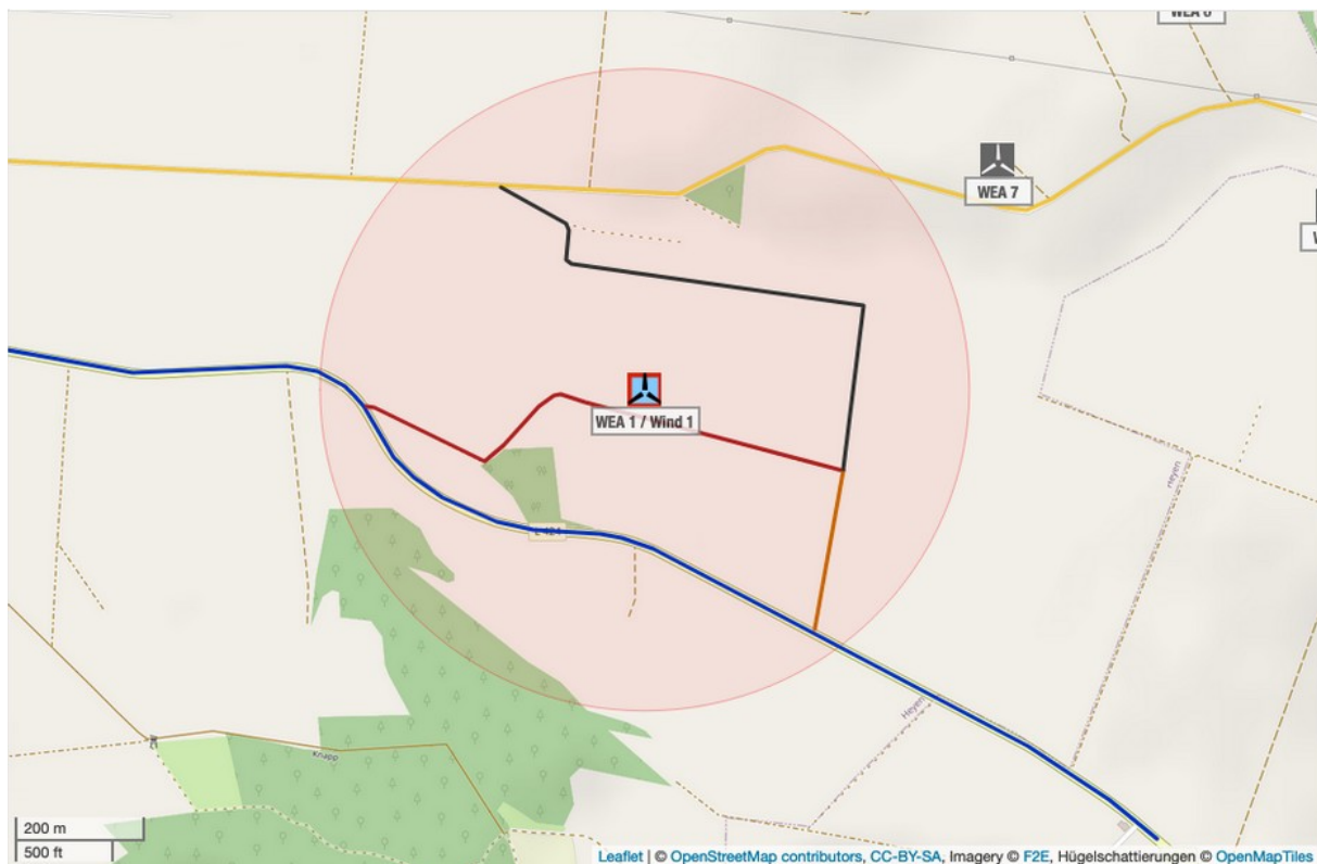
Abbildung 4.3.1: Potentieller Gefährdungsbereich der WEA 1 und Schutzobjekte am Standort Heyen (Karte /1.4/).
