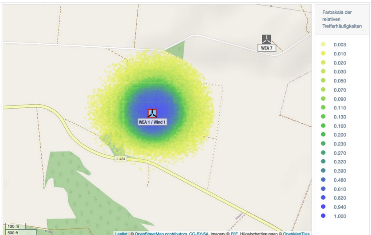
Abbildung A.1.1: Trefferhäufigkeiten von Eisstücken pro Rasterfläche (16m 2 ) und Jahr in der Umgebung der WEA 1 am Standort Heyen (Karte /1.4/).
