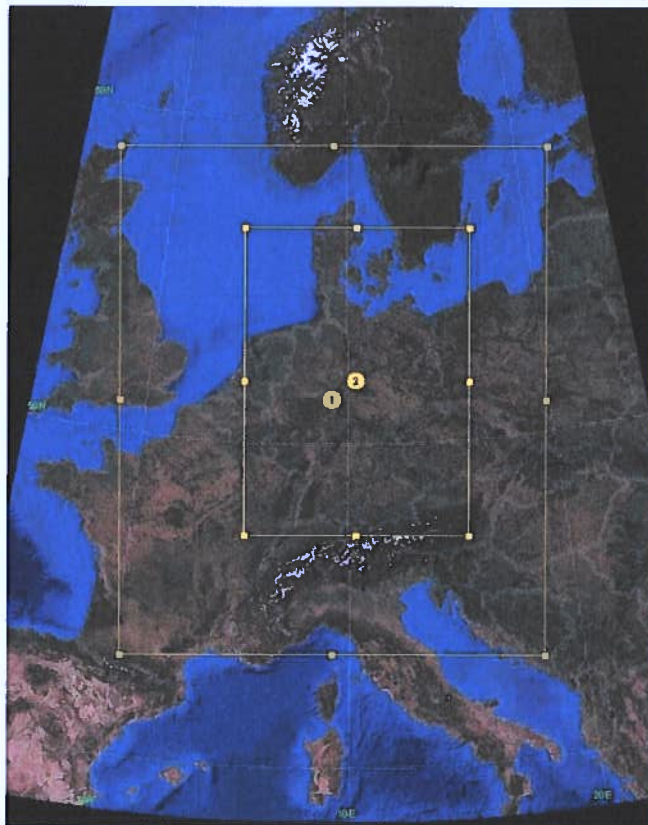
Abb. 2: Verschachtelte Domains der WRF Simulationen
