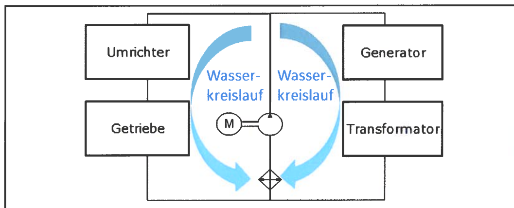
Abb. 3: Schematische Darstellung Kühlkreislauf
