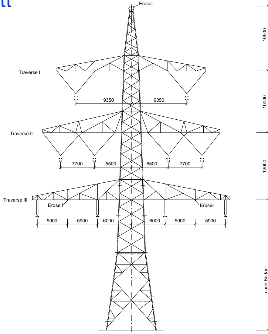
Tragmast T2-spez.; DA-4-DE-2015.2 Mast-Nr. C081
