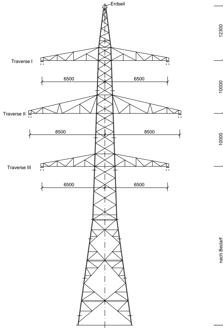
Winkelabspannmast WA 160; D-2-T-2014.2 Mast-Nr. C065, C070
