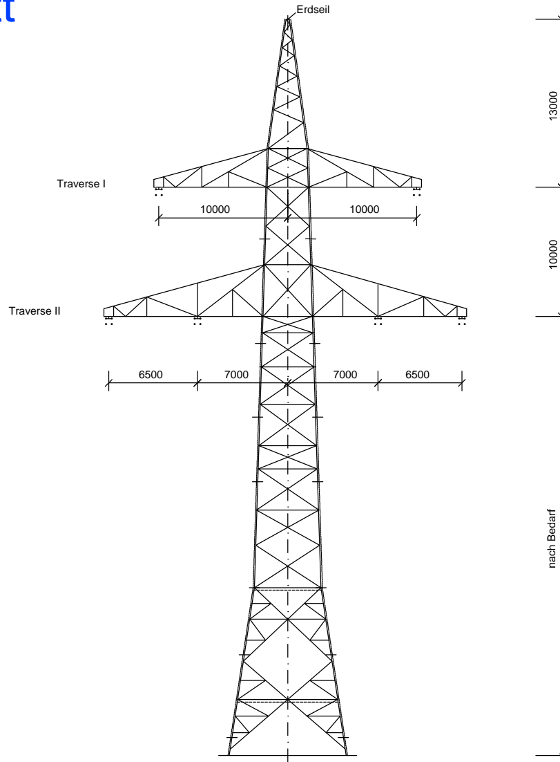
Winkelabspannmast WA 140; D-2-D-2013.1 Mast-Nr. C052, C056, C057
