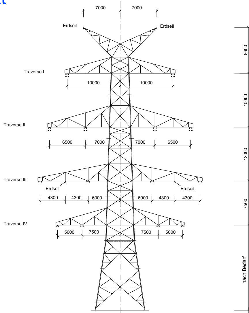
Winkelabspannmast WA 140; DAA-6-DEE-2014.1 Mast-Nr. C030, C031, C034, C035
