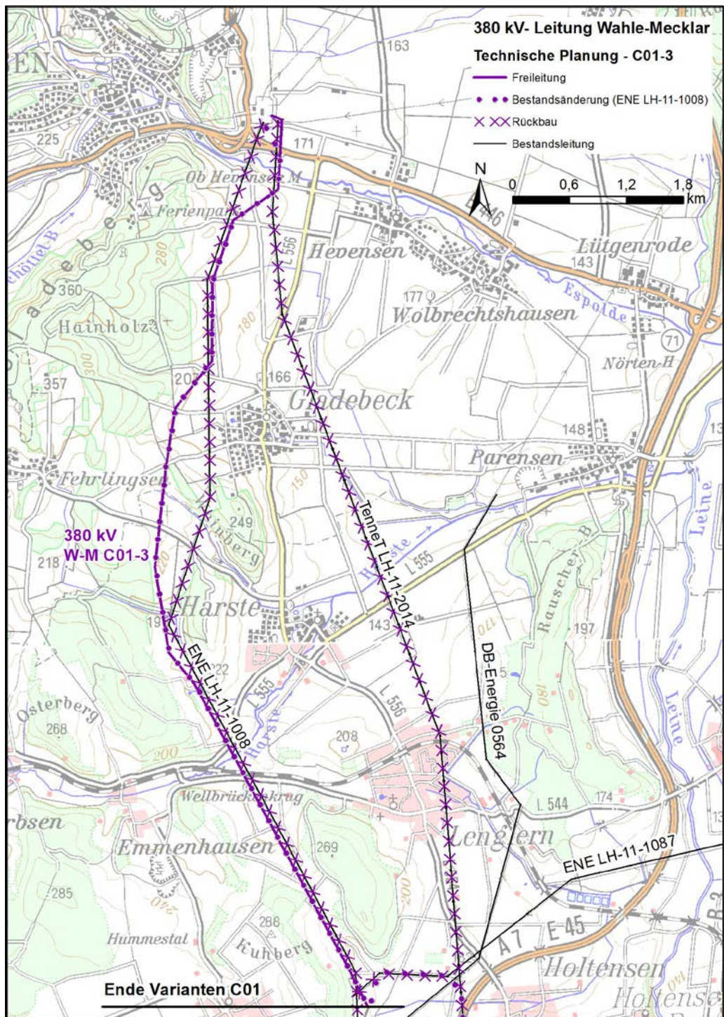
Abbildung 3: Technische Planung Variante C01-3
