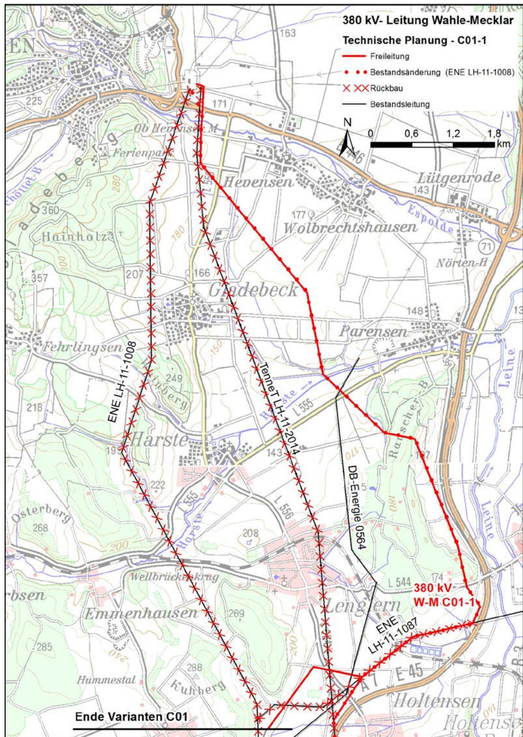
Abbildung 1: Technische Planung Variante C01-1
