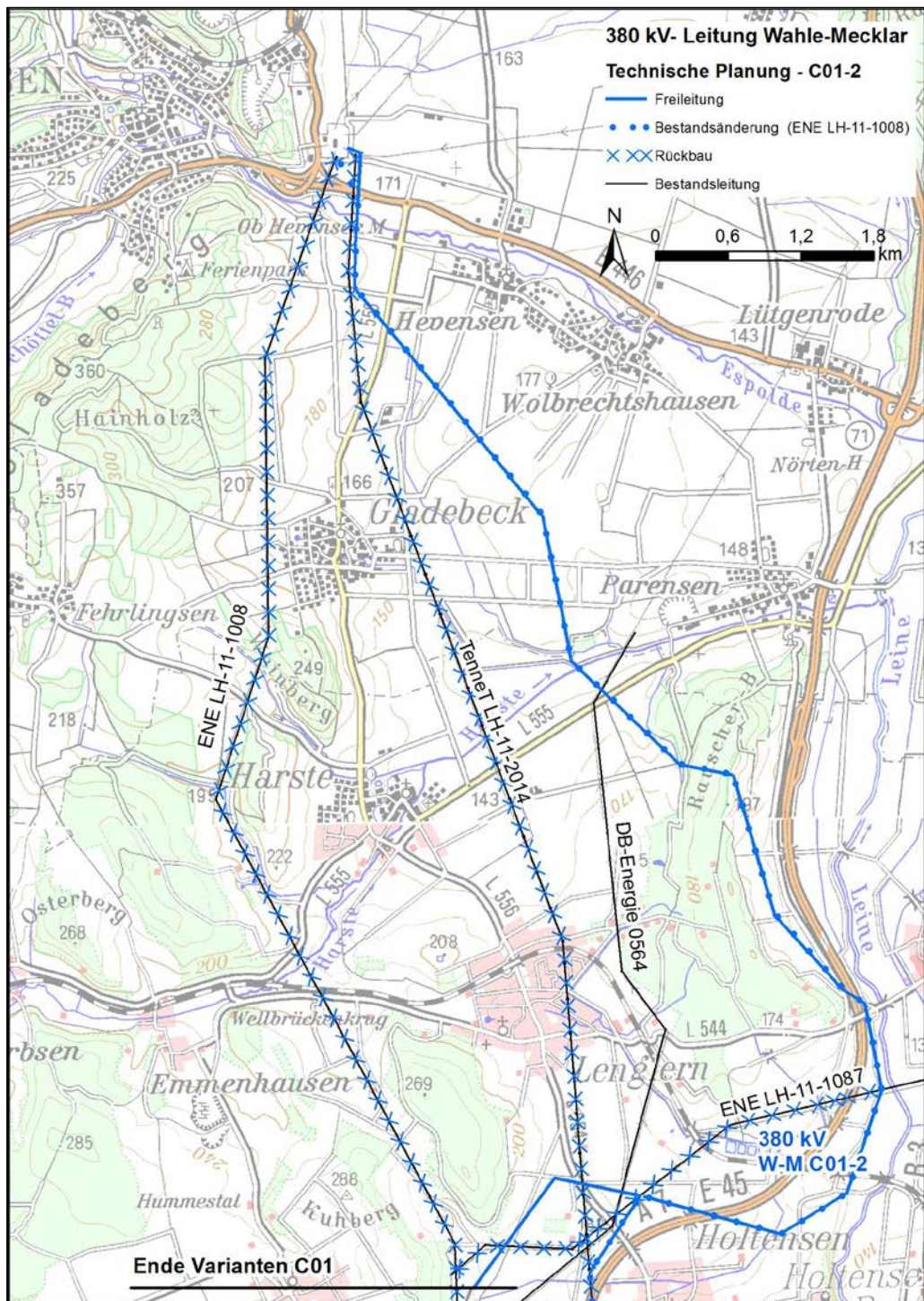
Abbildung 2: Technische Planung Variante C01-2
