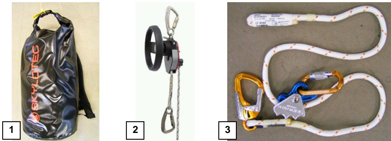
Abb. 6 Hauptbestandteile der Abseilausrüstung
