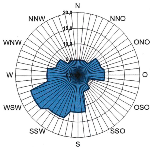
Abbildung 2: Relative Häufigkeit der Windrichtung am Standort Hollenstede (Fläche 18) in Prozent (Bezugshöhe 159,64m ü. Grund) /22/
