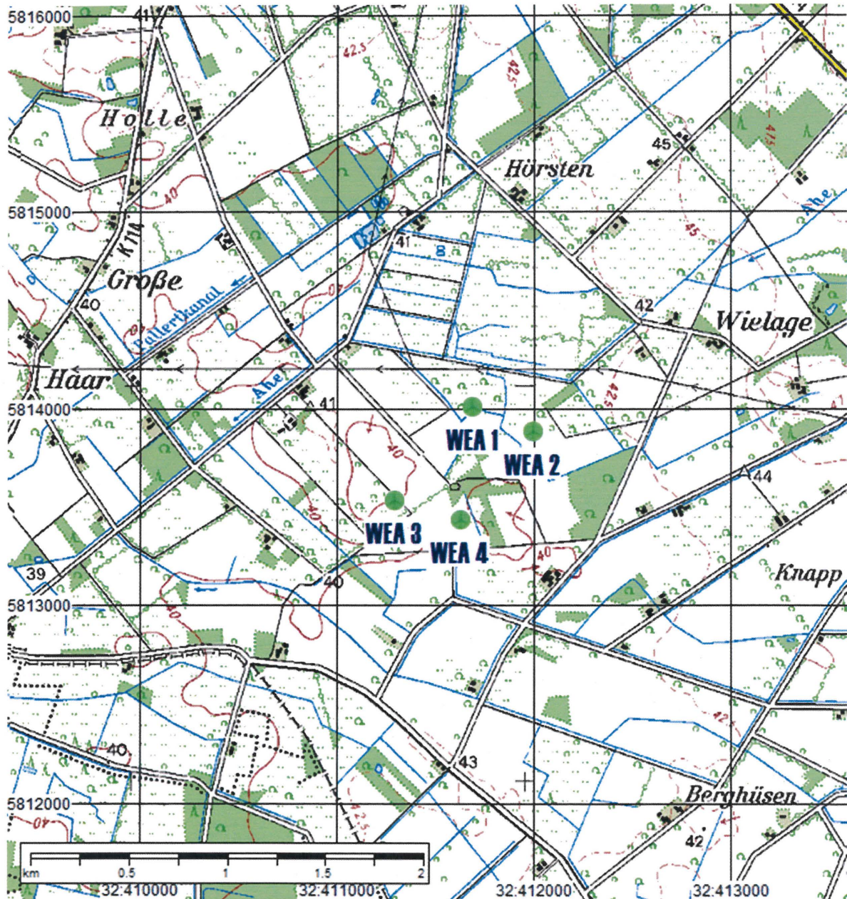
Abbildung 1: Lage des Windparks, Auszug topografische Karte 1:50.000 (vergrößerte Darstellung) /16/
