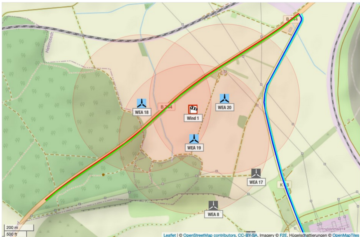
Abbildung 4.3.1: Potentielle Gefährdungsbereiche der WEA 18 - 20 und Schutzobjekte am Standort Helmstedt (Karte /1.4/).
