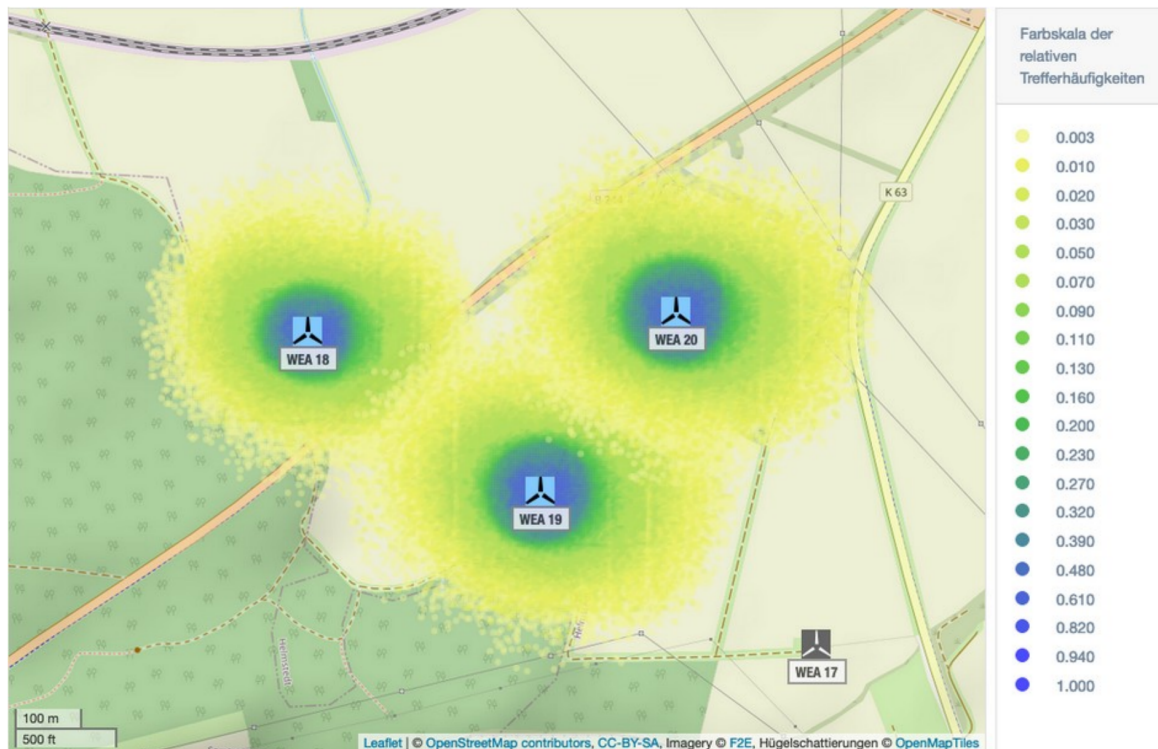
Abbildung A.1.1: Trefferhäufigkeiten von Eisstücken pro Rasterfläche (16m 2 ) und Jahr in der Umgebung der WEA 18 - 20 am Standort Helmstedt (Karte /1.4/).
