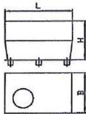
Bauform A Grundform ohne Nische
